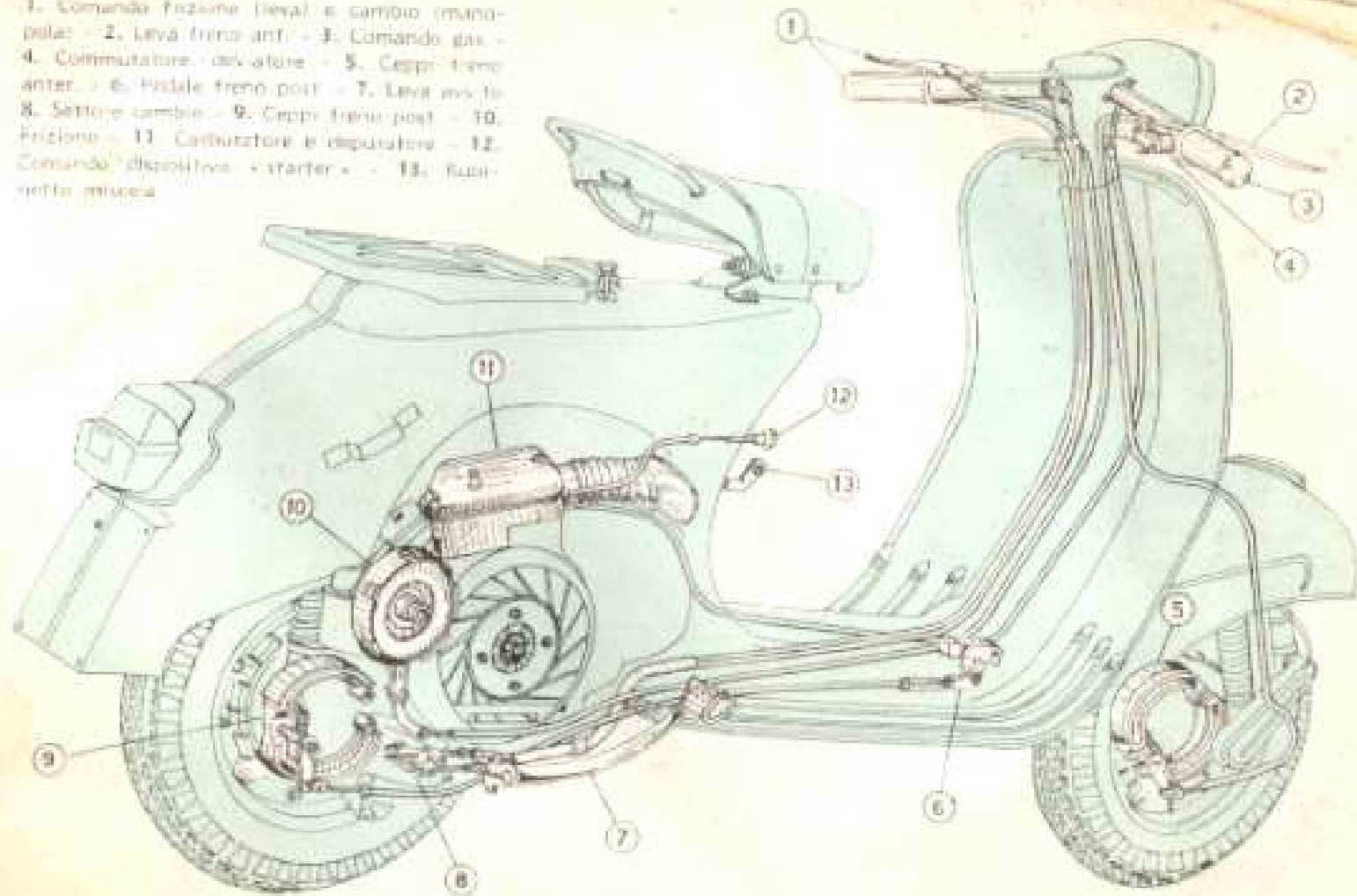
Fig. 2 - Installazione comandi e trasmissioni
