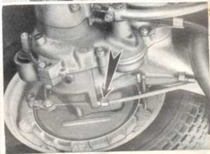
FIG. 17 - Registrazione dei freni
