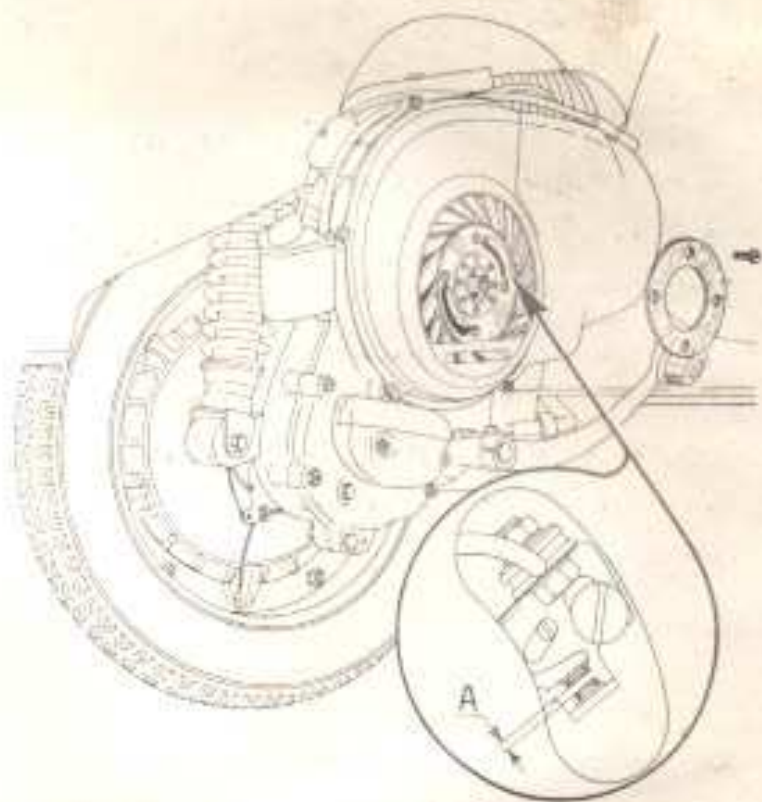
Fig. 22 - Registrazione puntine del ruttore
