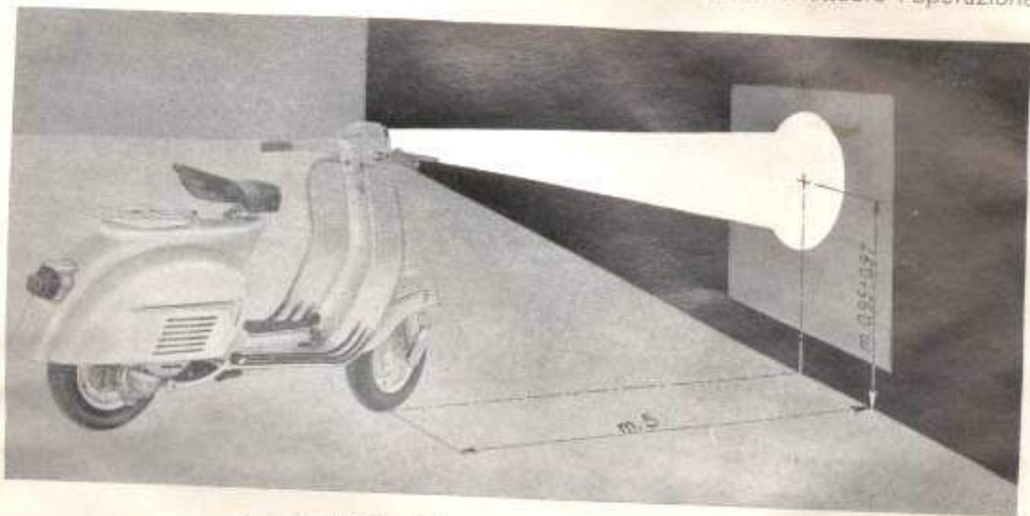
Fig. 21 - Schema orientamento proiettore
