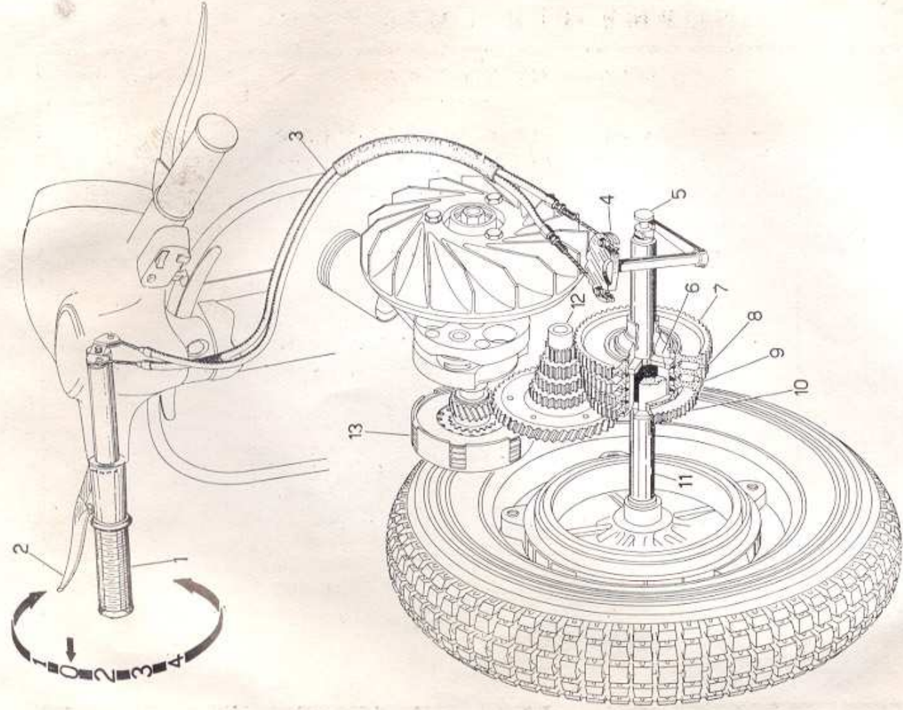
Fig. 15 - Schema del cambio
